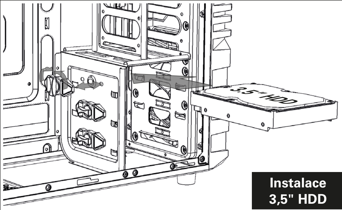
Instalace 3,5" jednotky
